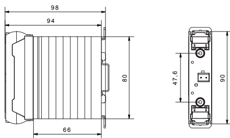
GNR Vorderansicht
