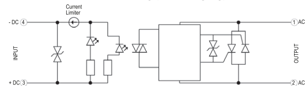
GNR Series 4-32 V DC Steuerung (Nulldurchgang)
